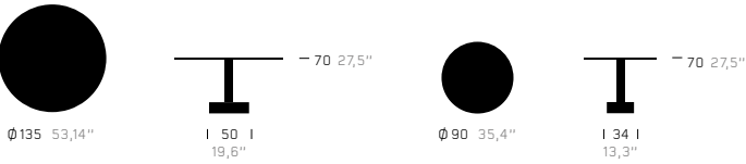
DINING TABLE Ø135 & Ø90 23772-00C-L1 / 56660-000-...
